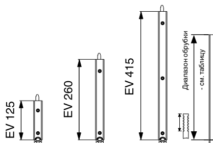
Концевые запоры для штульпового механизма
