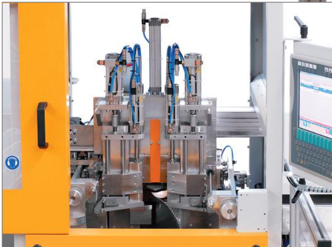
Модульное исполнение фиксаторов и пильного агрегата
